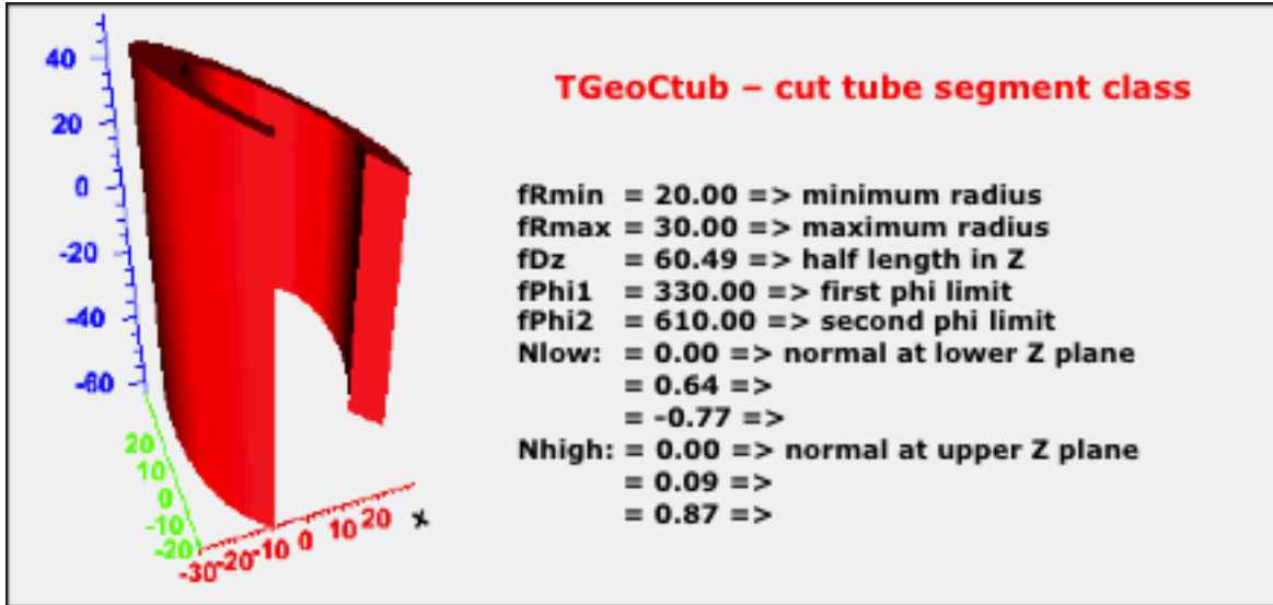
Figure 18.13: TGeoCtub Class
