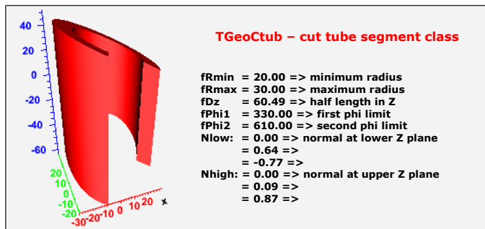
Figure 18-13 TGeoCtub Class
