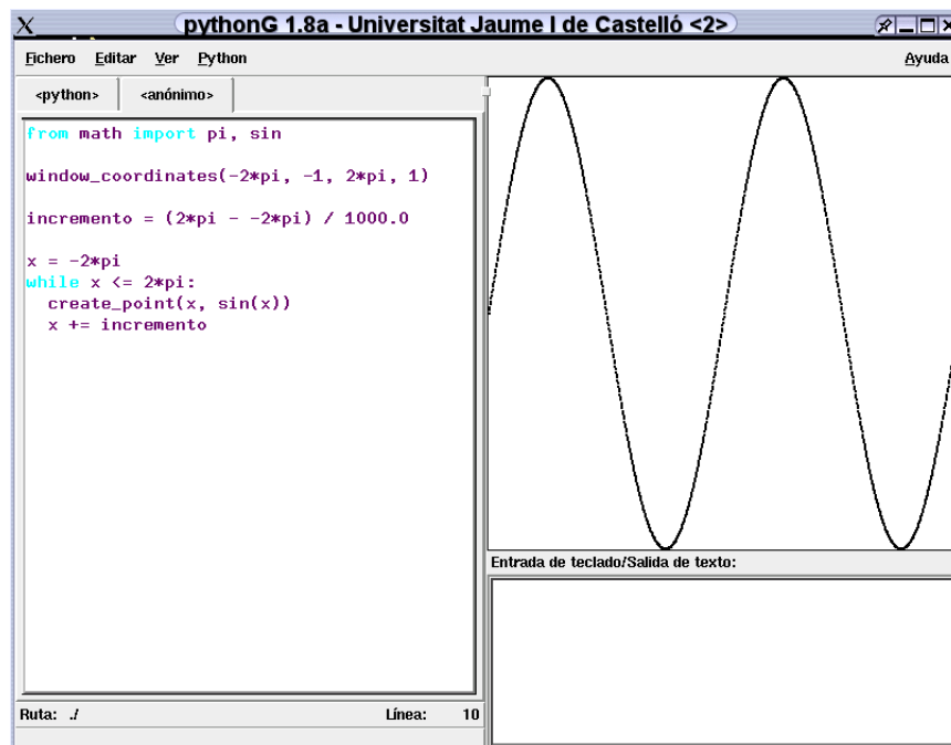
Figura 4.4: La función seno trazada con 1000 puntos.
