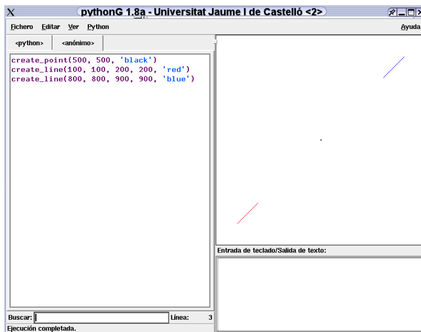
Figura 4.1: Programa prueba_grafica.py y su salida gráfica en el entorno PythonG.
