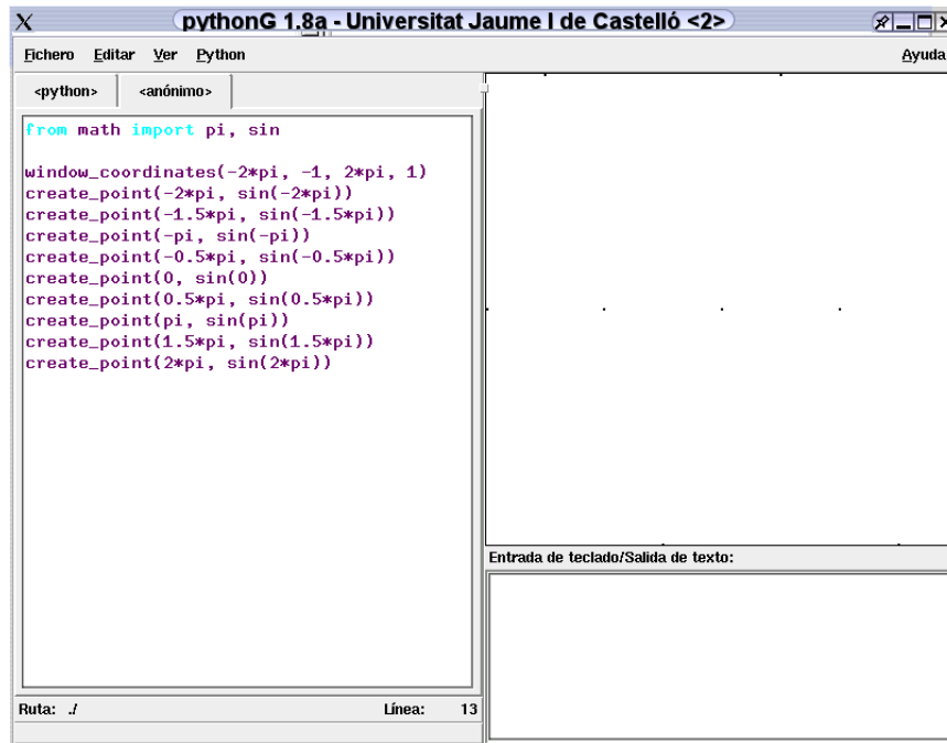
Figura 4.2: Primeras pruebas para dibujar la función seno.
